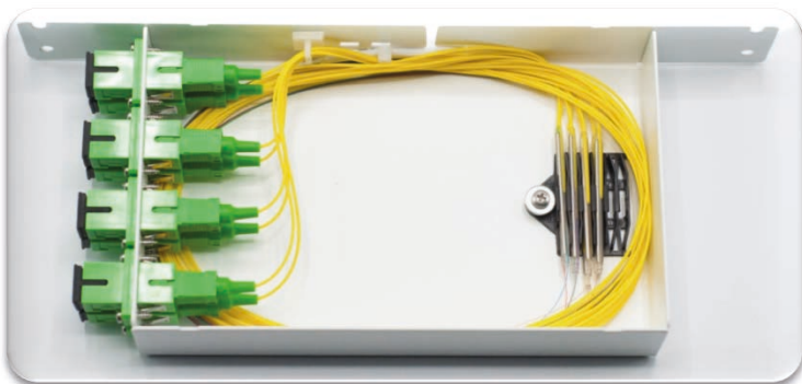
SCHEDA DI GIUNZIONE U.I.
