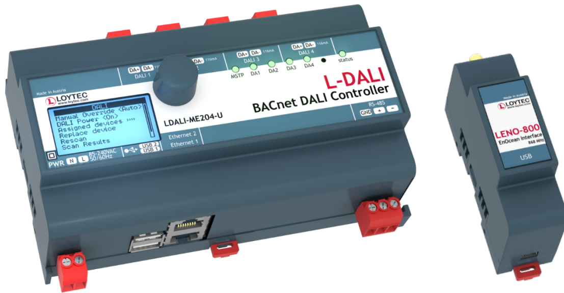
Interfaccia EnOcean
